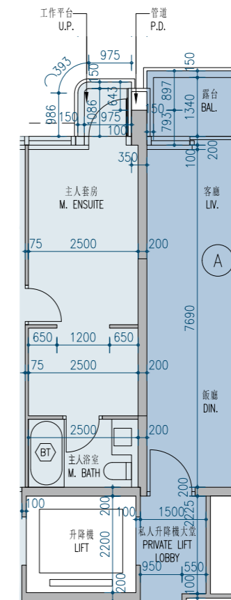
15/F-30/F Unit A & Unit B Part Plan 15樓至30樓 A單位及B單位之部分平面圖
