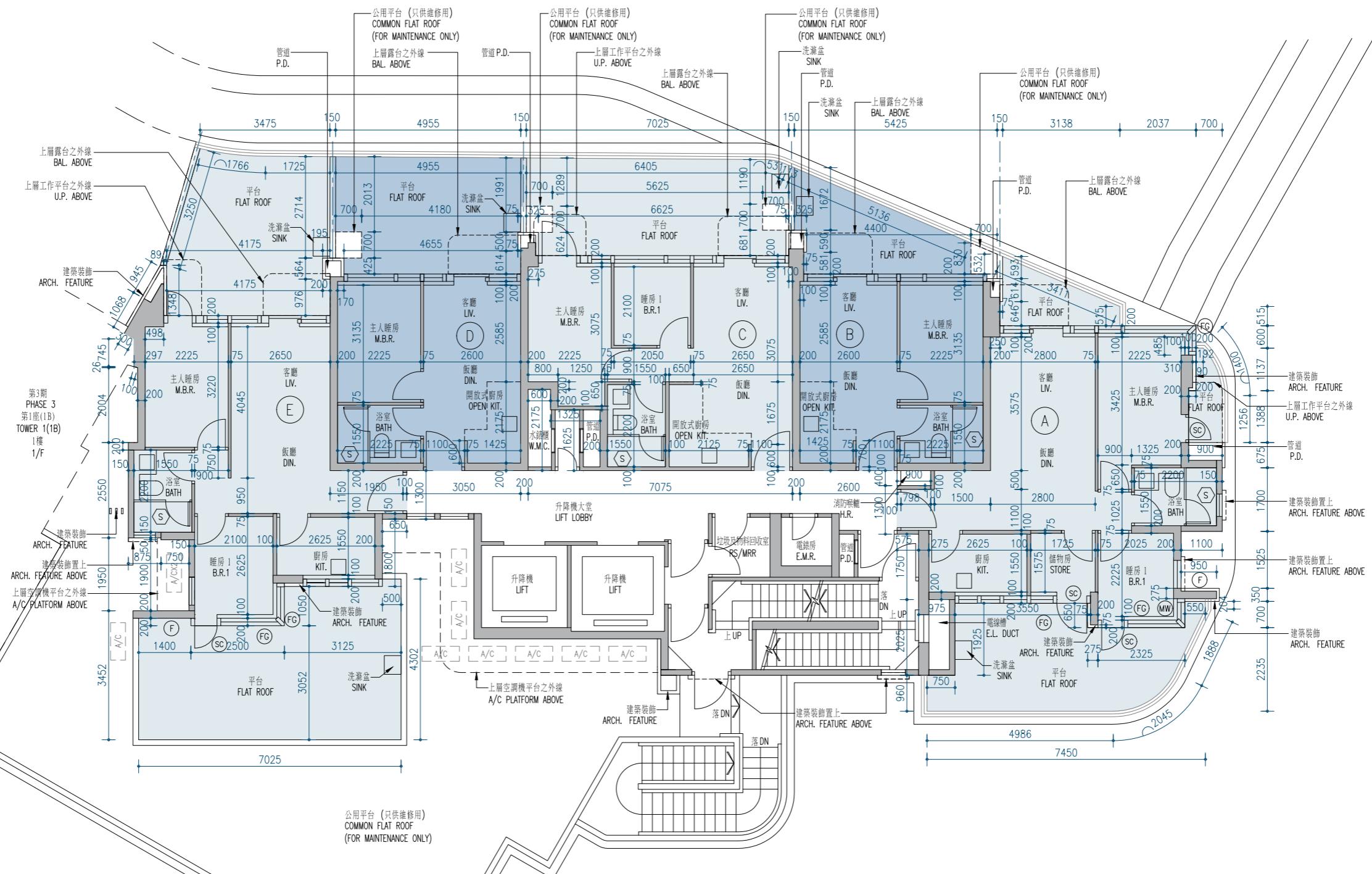
Phase 3 Tower 2 1/F Floor Plan 第3期 第2座 1樓樓面平面圖
